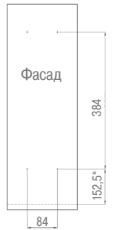
Присадочные размеры для установки фасада
