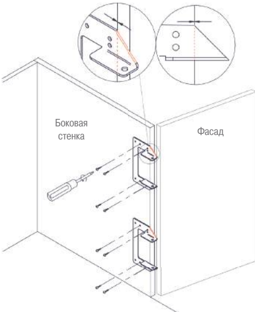
Монтаж креплений к боковине шкафа
