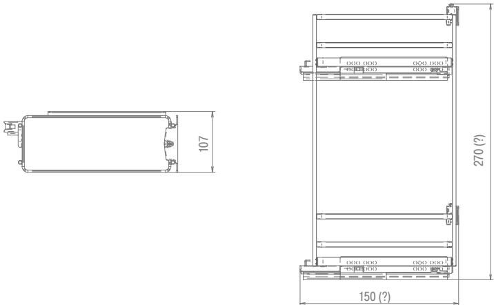
Габаритные размеры
