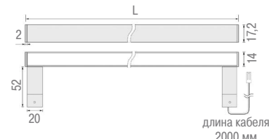
Установка светильника
