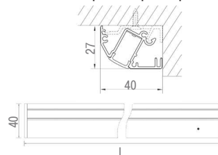
Габаритные размеры
