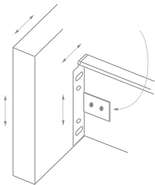
Эксцентриковая регулировка фасада
