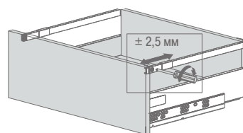
Регулировки для релинга
