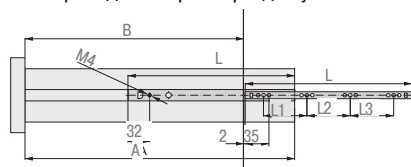
Присадочные размеры для установки направляющих
