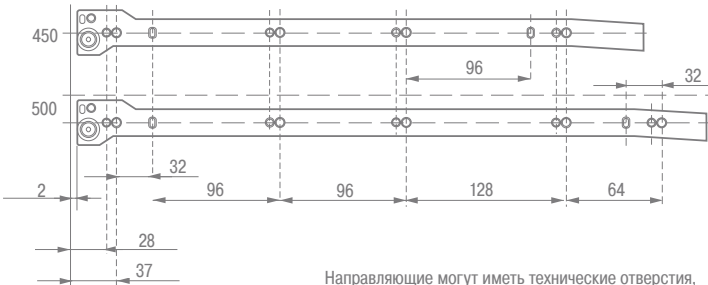
Присадочные размеры для установки направляющих
