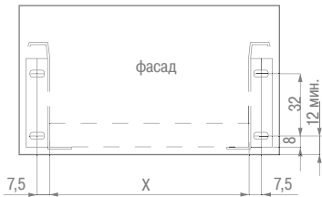
Присадочные размеры для сборки ящиков
