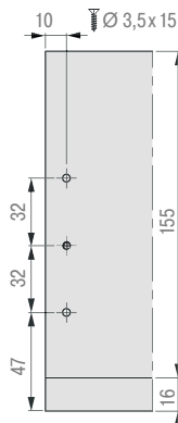
Размеры для установки направляющих полного выдвижения
