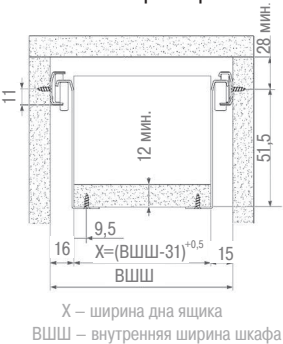
Размеры для раскроя дна ящика
