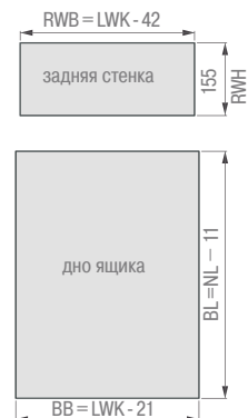
Размеры для установки направляющих полного выдвижения
