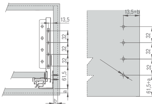
Присадочные размеры фасада
