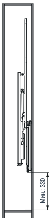
Установка справа
