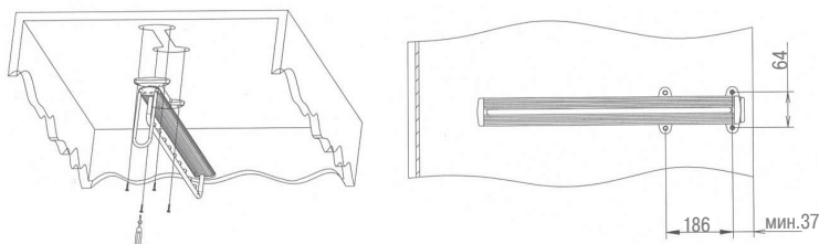
Присадочные размеры для установки держателя
