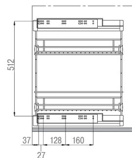
Присадочные размеры
